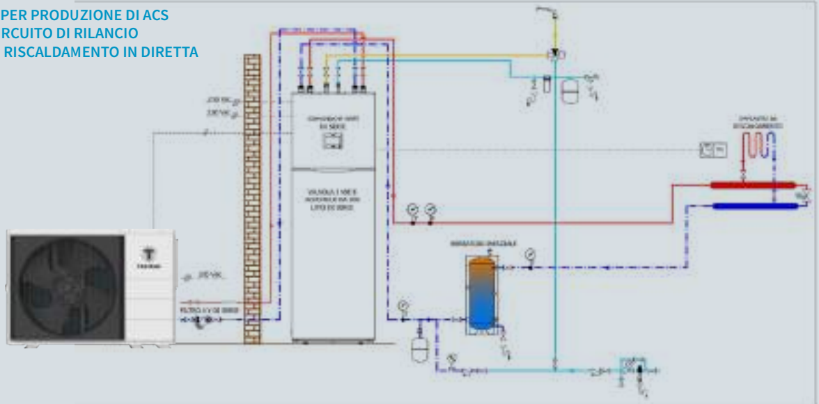
POMPA DI CALORE PER LA PRODUZIONE ACS INTEGRATA E PER LA GESTIONE DI UN CIRCUITO DIRETTO PER IL RISCALDAMENTO A MEDIA/ALTA TEMPERATURA E IL RAFFRESCAMENTO E UN CIRCUITO MISCELATO PER IL RADIANTE A PAVIMENTO IN BASSA TEMPERATURA
