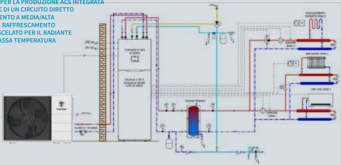
POMPA DI CALORE PER LA GESTIONE DI UN CIRCUITO DIRETTO PER IL RISCALDAMENTO CON I RADIATORI E PER IL RAFFRESCAMENTO CON DEI FAN COILS
